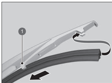
1 Prowadnica
