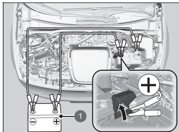
1 Zewnętrzny akumulator
