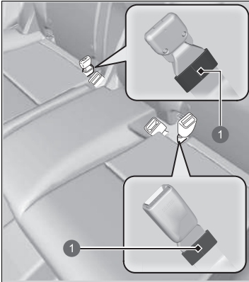
1 Uchwyt pasa
