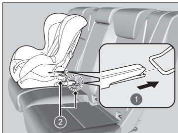
1 Sztywne złącze 2 Dolne mocowania
