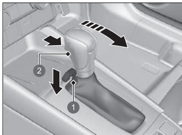
1 Szczelina zwalniania blokady dźwigni zmiany biegów
